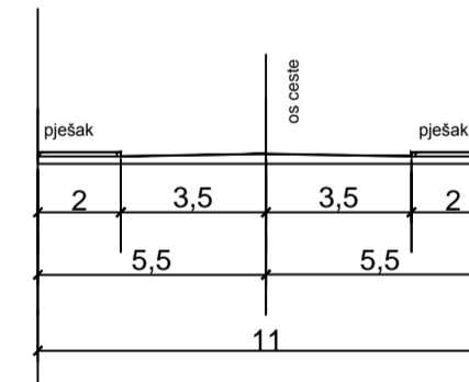
KARAKTERISTIČAN POPREČNI PRESJEK "A" Mj 1:200
