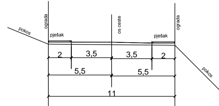
KARAKTERISTIČAN POPREČNI PRESJEK "B" Mj 1:200
