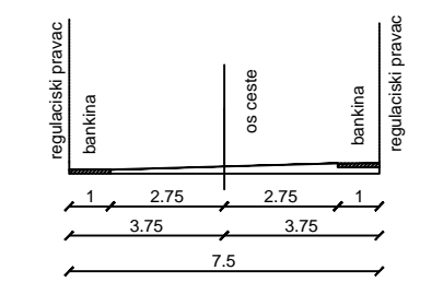
KARAKTERISTIČAN POPREČNI PRESJEK B - B, MJ. 1:200
