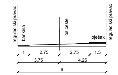
KARAKTERISTIČAN POPREČNI PRESJEK A - A, MJ. 1:200
