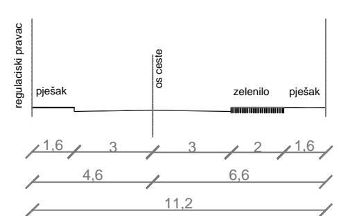
KARAKTERISTIČAN POPREČNI PRESJEK B-B
