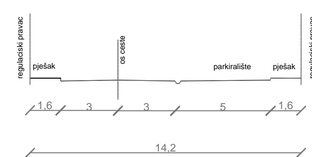
KARAKTERISTIČAN POPREČNI PRESJEK C-C
