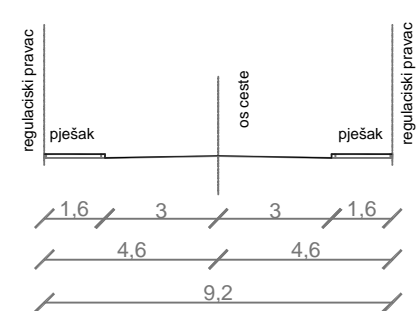
KARAKTERISTIČAN POPREČNI PRESJEK A-A
